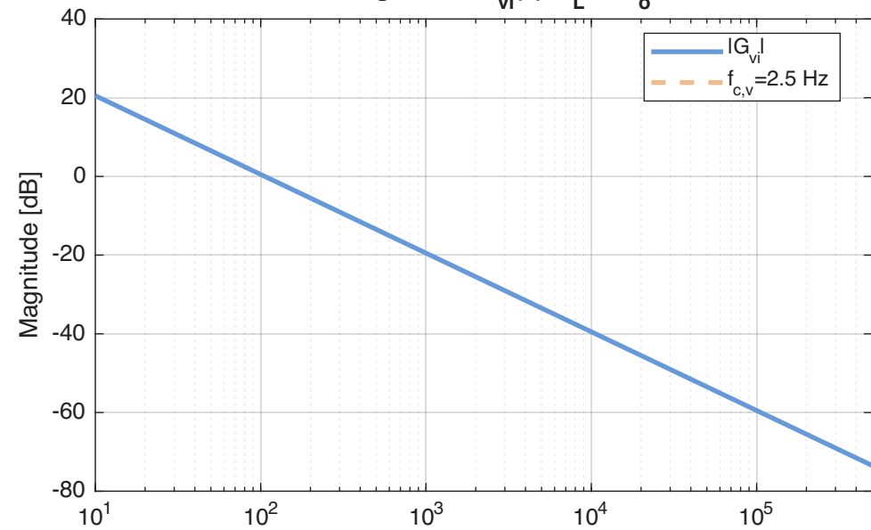
Voltage Plant G_{vi}(s) : i_L \rightarrow v_o
